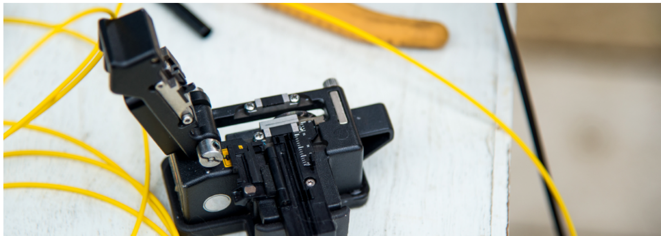
RCLV-100CRH | CORTADORA DE PRECISIÓN PARA FIBRA ÓPTICA
